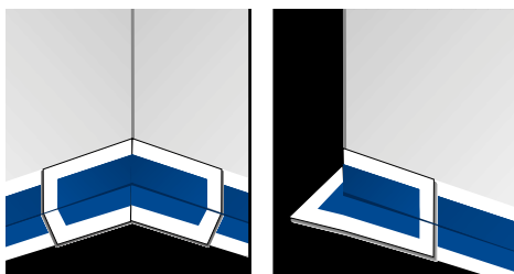
Postavljanje gotovog ugla od 90°
